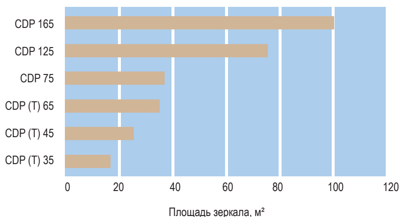
ДИАГРАММА БЫСТРОГО ПОДБОРА ОСУШИТЕЛЕЙ
